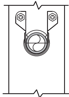
Hanger - Wood Stud
